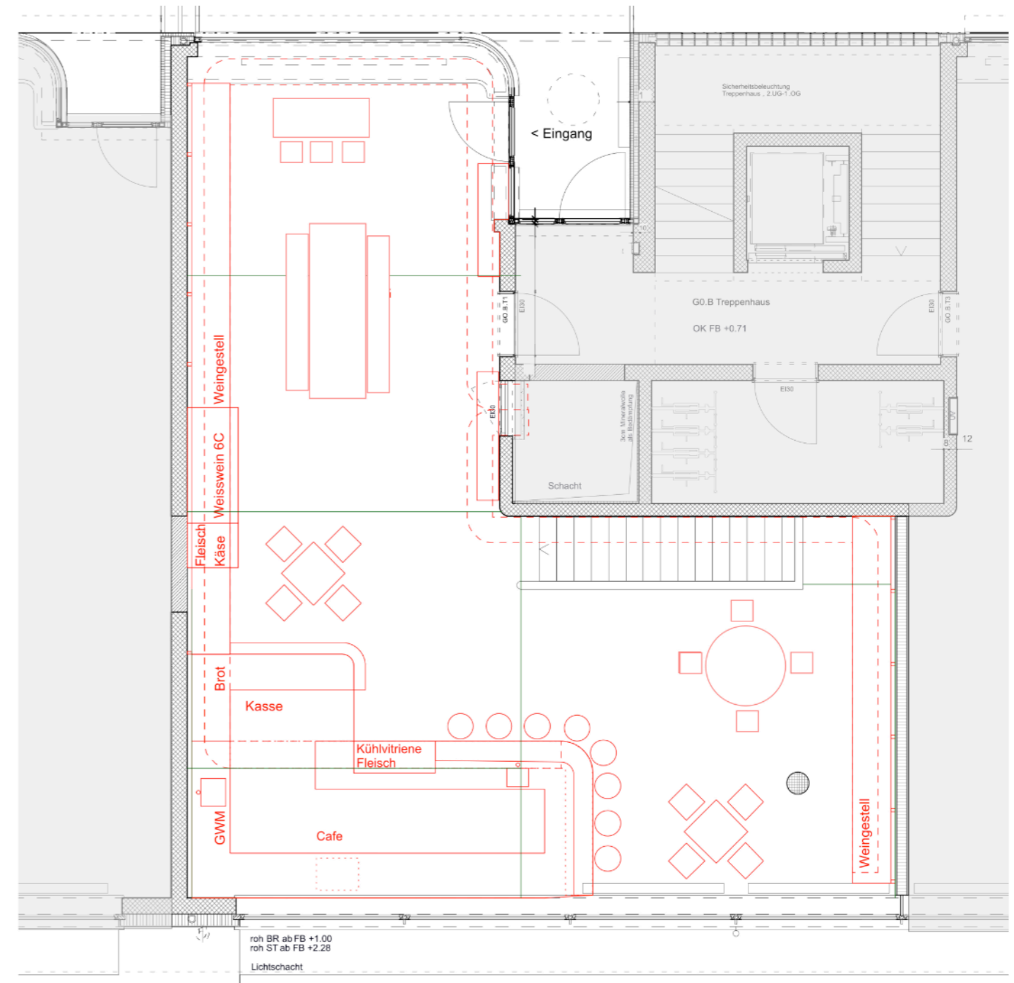
Erdgeschoss
